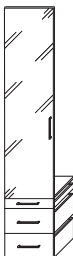
Spiegeltür, mit drei Schubkästen und einem Konstruktionsboden Maße: B/H 45/224 cm
